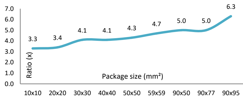
圖表 9：封裝尺寸效益比較
