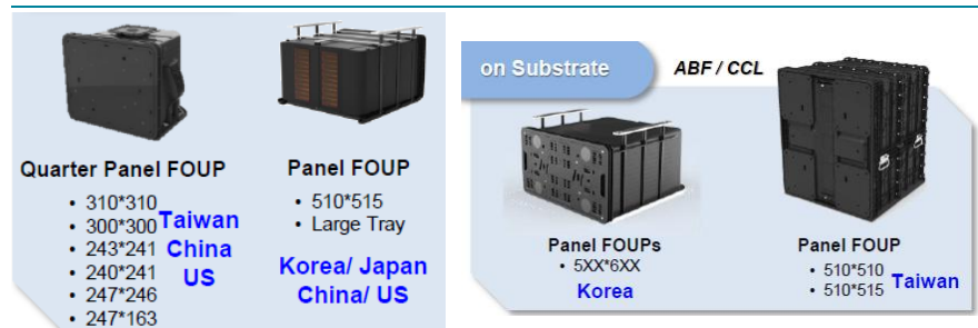
圖表 8：家登面板級封裝載具產品線
